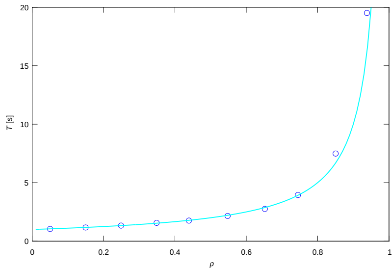
Slika 3.9: Prosečno zadržavanje korisnika u sistemu.
