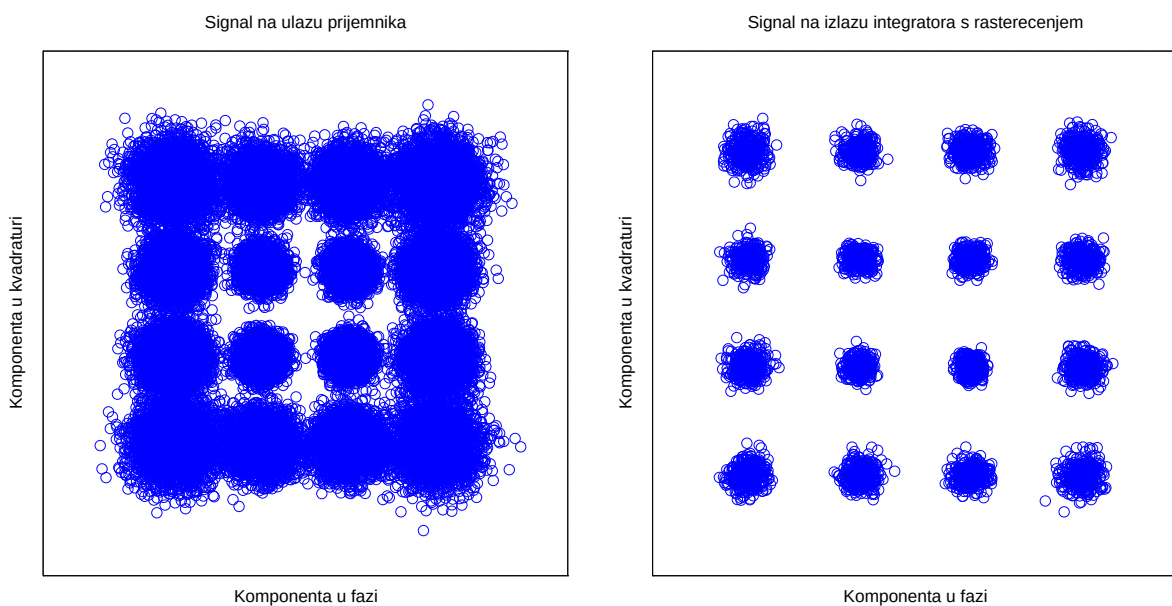
Slika 12.2: Konstelacioni dijagrami signala.
