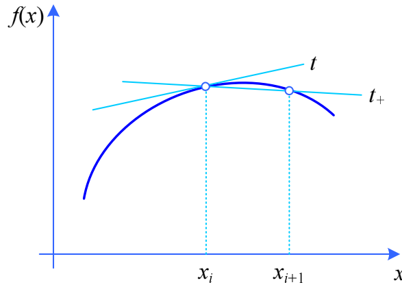
Slika 4.1: Diferenciranje unapred.
