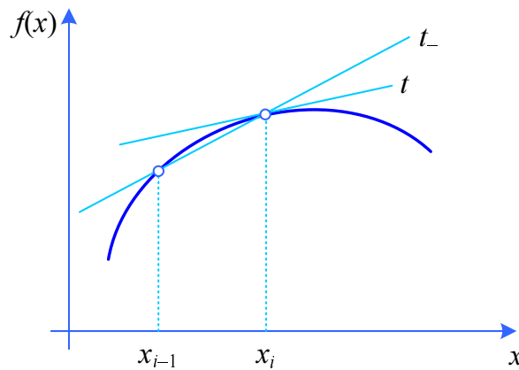
Slika 4.2: Diferenciranje unazad.
