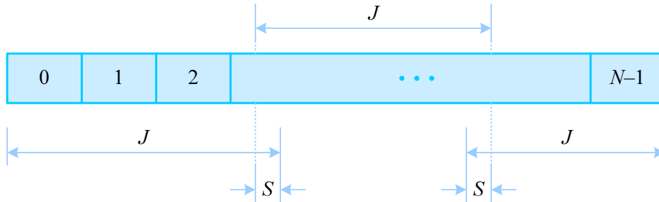
Slika 6.4: Ocena spektralne gustine srednje snage signala Welchovim postupkom.
