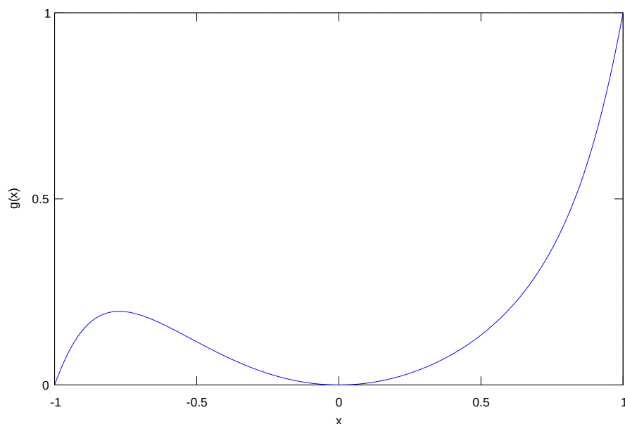
Slika 5.3: Grafik podintegralne funkcije.
