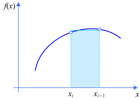
Slika 4.6: Centralno integriranje.
