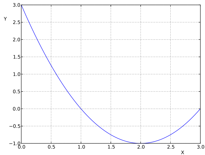
Slika 2.2: Grafik preslikavanja.
