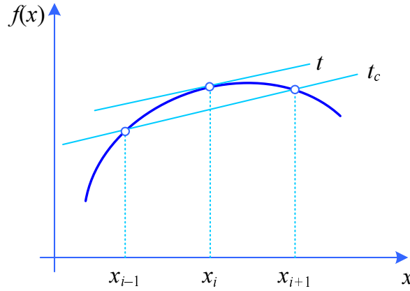
Slika 4.3: Centralno diferenciranje.
