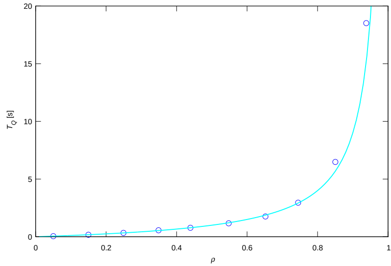
Slika 3.8: Prosečno trajanje čekanja.
